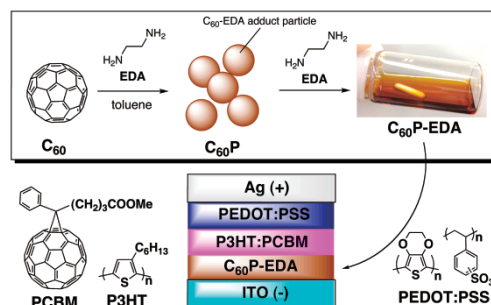
図1 フラーレン-ジアミン付加体をバッファ層に用いた有機薄膜太陽電池
